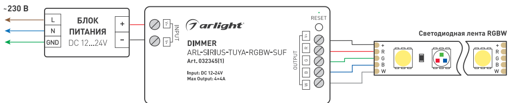
Рисунок 2. Пример схемы подключения диммера ARL-SIRIUS-TUYA-RGBW-SUF
