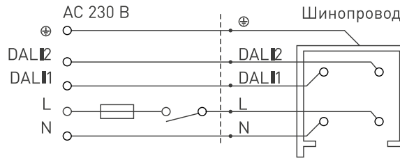
в) 1 фаза, 1 нагрузка, AC 230 В, 16 А, 1x3,7 кВА
