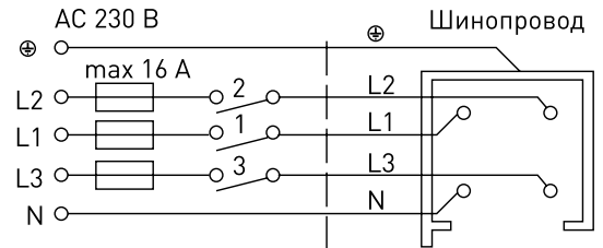
б) 3 фазы, 3 нагрузки, AC 230 В, 16 А, 3x3,7 кВА
